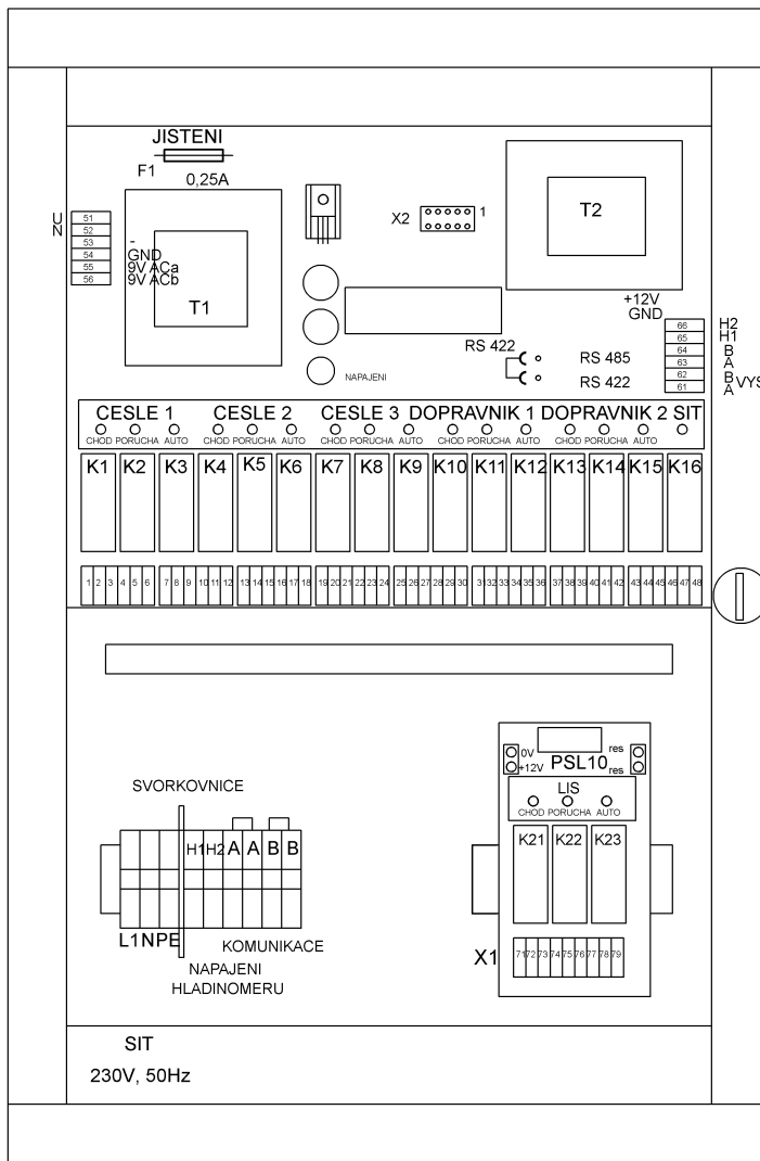
ZAPOJENI KONEKTORU X1
